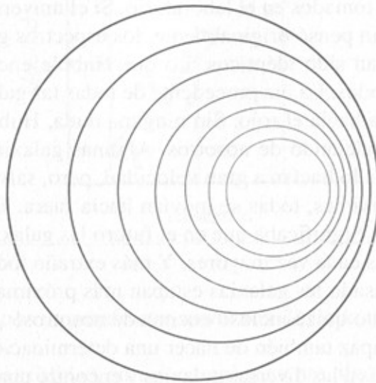
ondas procedentes de una fuente que se mueve hacia la derecha
