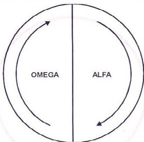
Figura 3 El Dios Padre-Madre La salida y la entrada de los ciclos de Alfa y Omega
