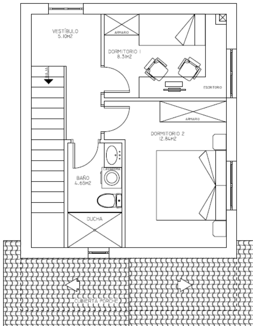
PLANTA PRIMERA
