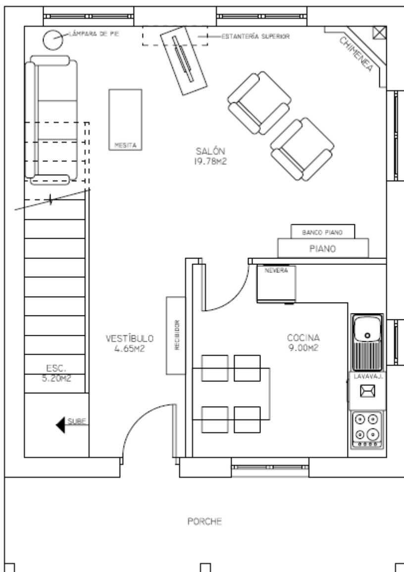
PLANTA BAJA
