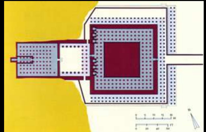
Planta del templo mortuario
