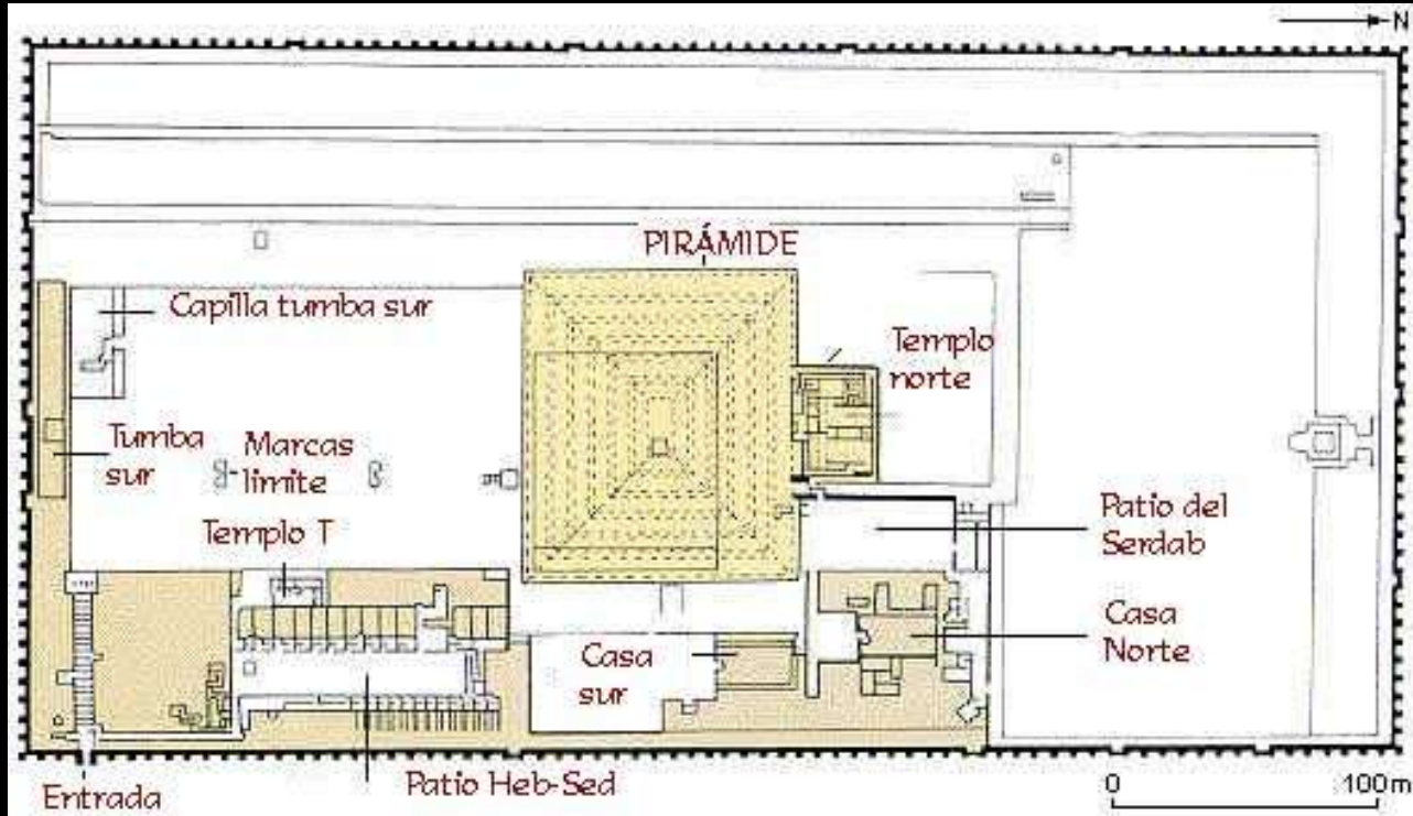
Planta conjunto Sakkara
