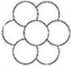
El Huevo de la Vida - Ley de Octava para la Música
