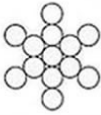
La Fruta de la Vida - Desdoblamiento de la ley de 13
