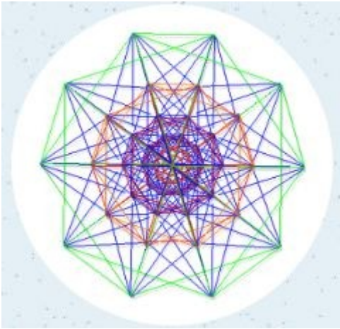
Estrella Madre - 5 sólidos platónicos autocontenidos (imagen por Heartcoherence- Dan Winter) .
