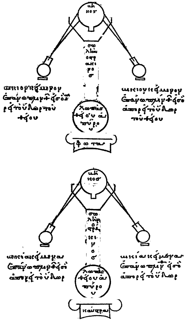
FIGURES 14 et 14 bis. — Alambic à deux récipients ( dibicos ) Réduction aux 2/3.
