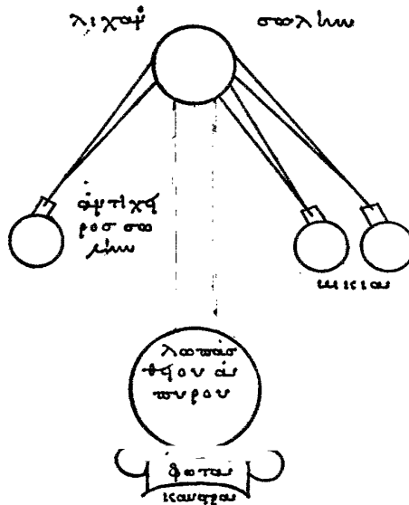
FIGURE 15. — Alambic à trois récipients ( tribicos ). Réduction aux 2/3.
