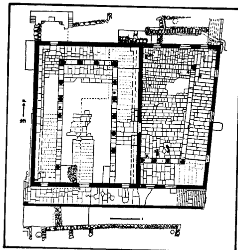
Fig. 9: Planta del edificio de la sinagoga. Se componía de tres partes. A la izquierda, la sala de oración, con 16 columnas interiores.
