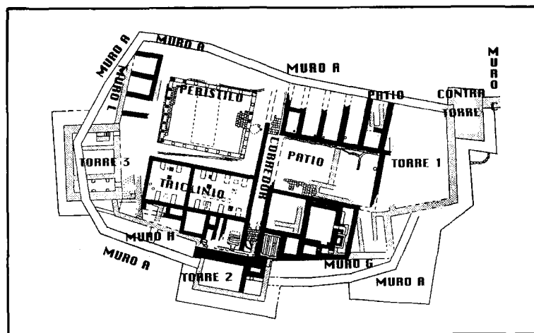
Fig. 3: La fortaleza-palacio de Maqueronte, construida sobre la cima de la montaña. Tenía 100 m de largo y 60 m de ancho. Una fuerte muralla (muro A) la protegía en caso de ataque. Estaba dividida en dos secciones por un corredor central. A la derecha de él estaban las termas. A la izquierda, el comedor, frente a un amplio patio de columnas. Cuatro torres de 30 m de altura la defendían.
