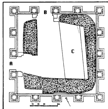
Fig. 4: Planta de la tumba de la Virgen María según las excavaciones. La roca de la pequeña cámara sepulcral quedó encerrada en una construcción de columnas de la época de las cruzadas. La entrada principal (A) tiene 1,43 m de altura. La otra (B) sólo 1,24 m, por lo que hay que inclinarse, tanto para ingresar como para salir. En el interior, cubierto por un vidrio, se puede ver el banco de piedra (C) donde los apóstoles recostaron el cuerpo de María, y de donde ella fue asunta a los Cielos.
