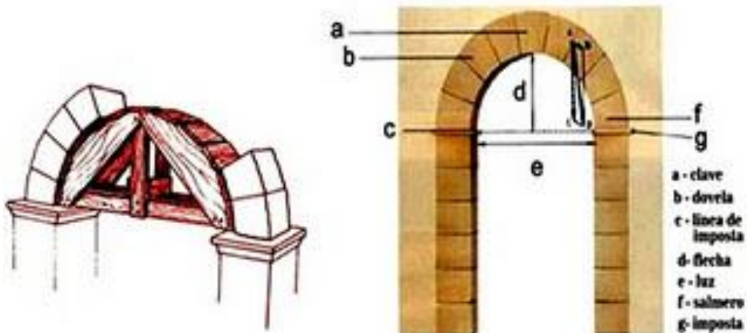
Partes que componen al Arco de Medio Punto, en la Arquitectura
