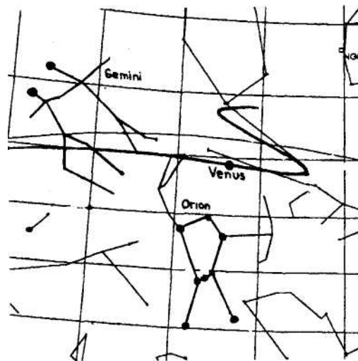
Figura 31 · Venus hará un giro planetario retrógrado a la derecha, encima de Orión, en la primavera y verano del año 2012. Este es el código astro-nómico OPUESTO al anterior. Señala un cambio catastrófico en los campos magnéticos del Sol y de la Tierra.
