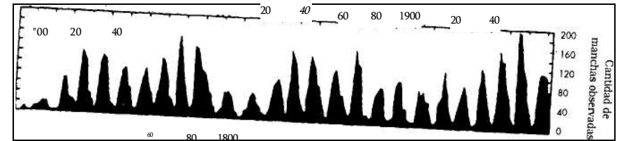
El ciclo (aproximado) de las manchas solares de 11^{1/2} años, de la observación efectuada desde 1680.
