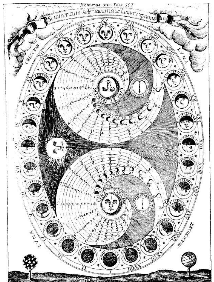
El ciclo Lunar de XXVIII dias (según Kircher)
