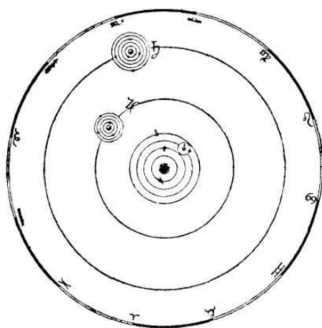
Fig. V.- Sistema de Copérnico. (El Sol está en el centro)
