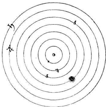
Fig. VI.- Sistema de Tolomeo. (La Tierra está en el centro)
