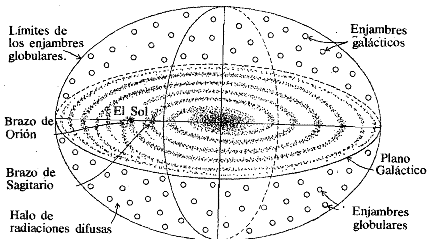
Perspectiva de la Galaxia El «huevo cósmico» de la Galaxia
