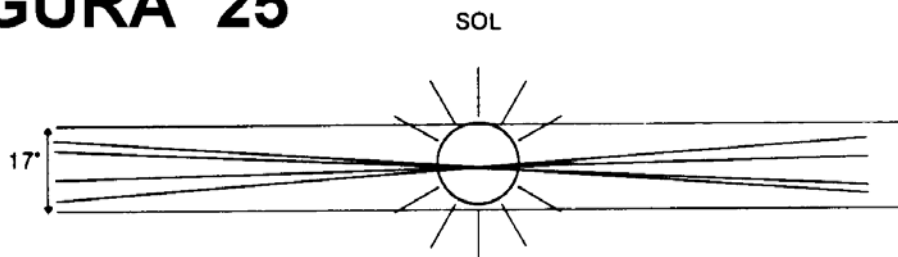
FIGURA 25 LAS ORBITAS ASTRONOMICAS DE LOS PLANETAS SE SEPARAN POCO
