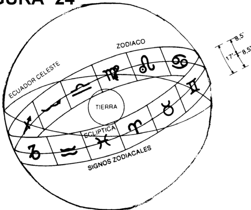
FIGURA 24 ZODIACO Y ANTERIORES
