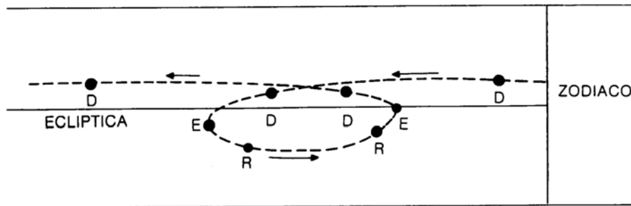
FIGURA 36 RIZO APARENTE DE UN PLANETA
