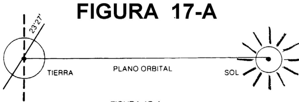
FIGURA 17-A INCLINACION DEL EJE TERRESTRE RESPECTO A SU PLANO ORBITAL
