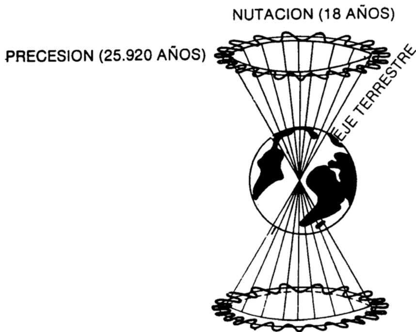
FIGURA 34 NUTACION Y PRECESION SIMULTANEAS
