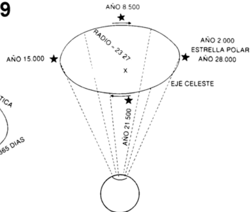
FIGURA 29 DESPLAZAMIENTO DEL POLO N. CELESTE EN EL CIELO: ACTUALMENTE APUNTA A LA ESTRELLA POLAR
