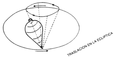
FIGURA 27 MOVIMIENTO DE PEONZA (TROMPO) DEL EJE TERRESTRE
