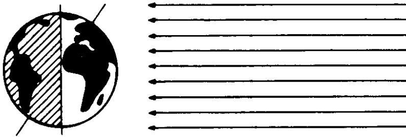
FIGURA 15 EL DIA Y LA NOCHE
