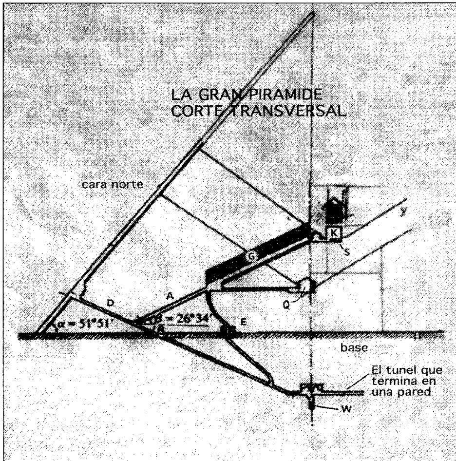
Corte transversal de la Gran Pirámide:
