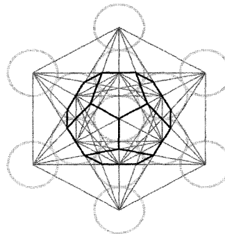
Dodecaedro
